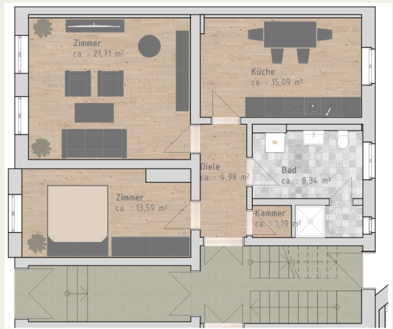
Abb. 02 · Wohnung Erdgeschoss links · Grundriss schematisch, nicht maßstabsgetreu
